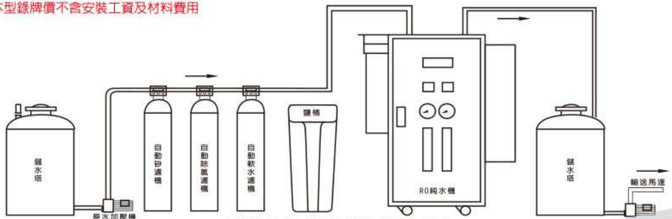
RO純水機安裝示意圖
